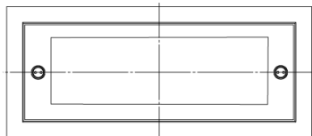
Dimensions d'encastrement 310
