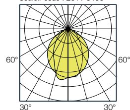
Couloir code : 2011 0400
